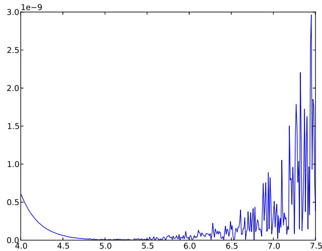
FIGURE 1 – Graphe de l'erreur pour la dérivation numérique en fonction du pas h = 10^{-y}
