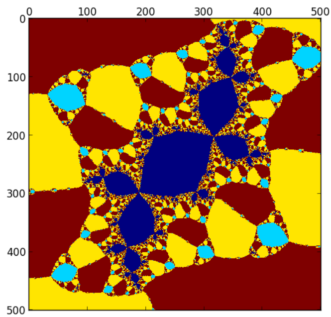
FIGURE 4 – Zoom sur le lapin de Douady
