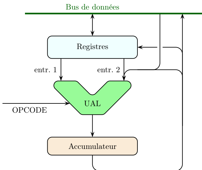
FIGURE 2.3 – Schéma d'une unité de traitement
