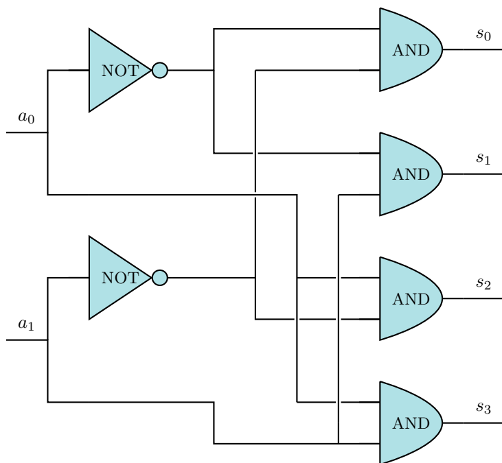
FIGURE 2.7 – Décodeur d'adresses sur 2 bits
