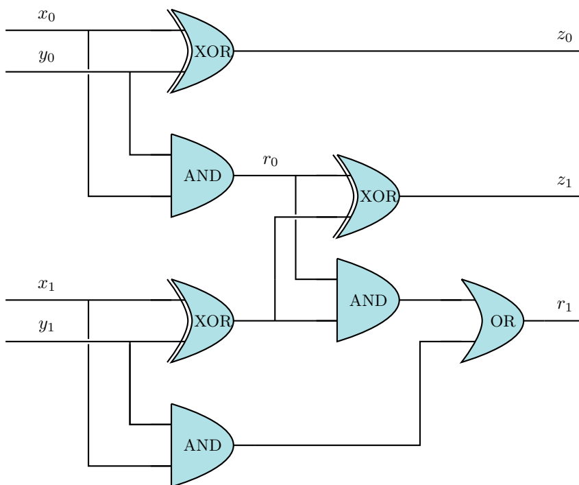
FIGURE 2.5 – Schéma logique d'un additionneur à 2 bits
