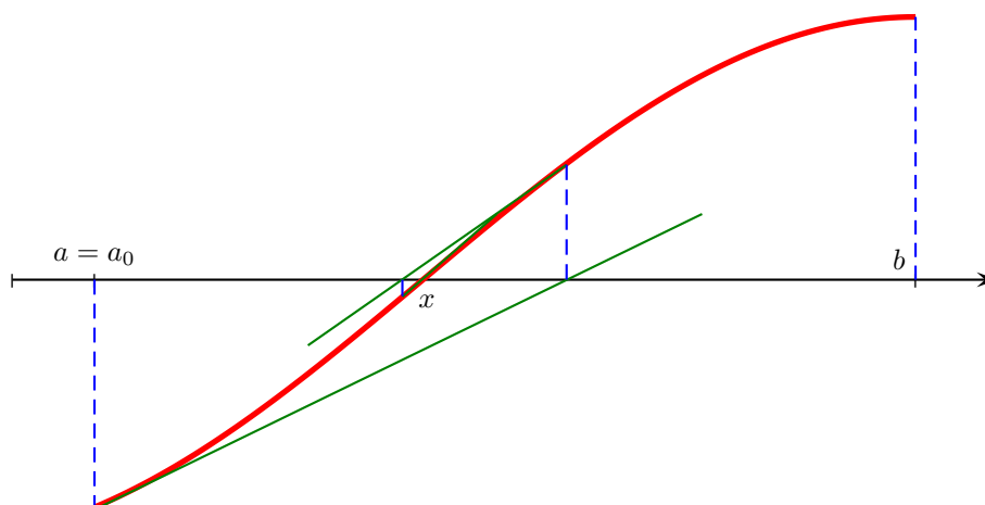
FIGURE 7.3 – Méthode de Newton
