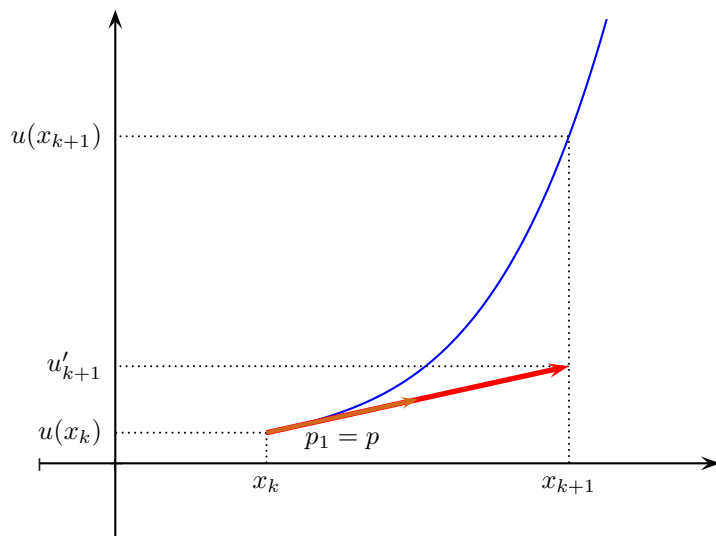
FIGURE 8.4 – Runge-Kutta d'ordre 1
