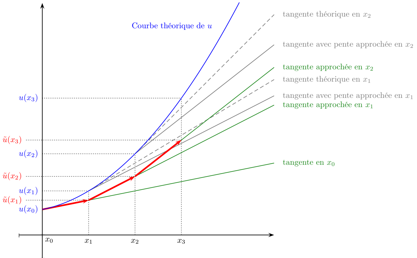
FIGURE 8.1 – Méthode d'Euler
