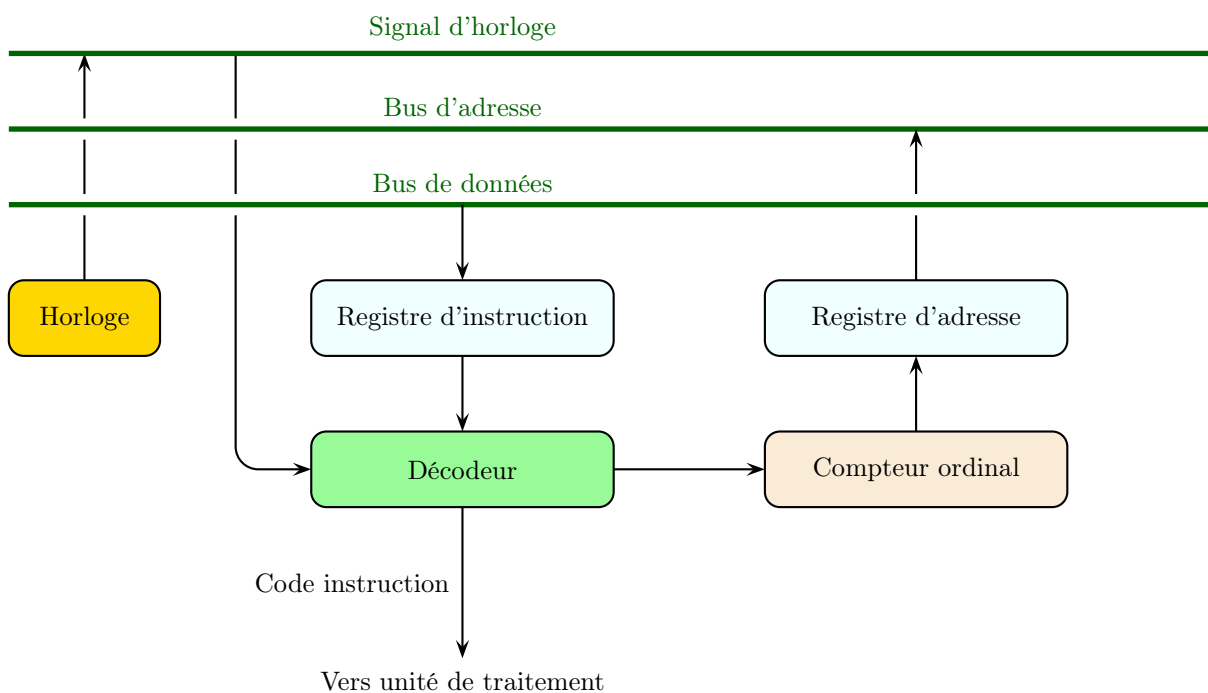
FIGURE 2.4 – Schéma d'une unité de contrôle
