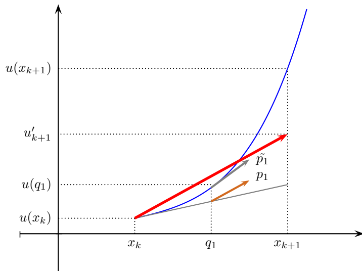
FIGURE 8.5 – Runge-Kutta d'ordre 2
