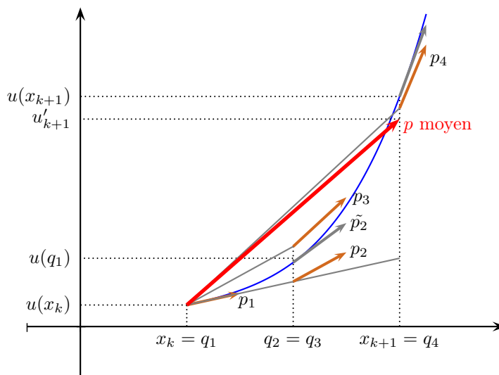
FIGURE 8.6 – Runge-Kutta d'ordre 4
