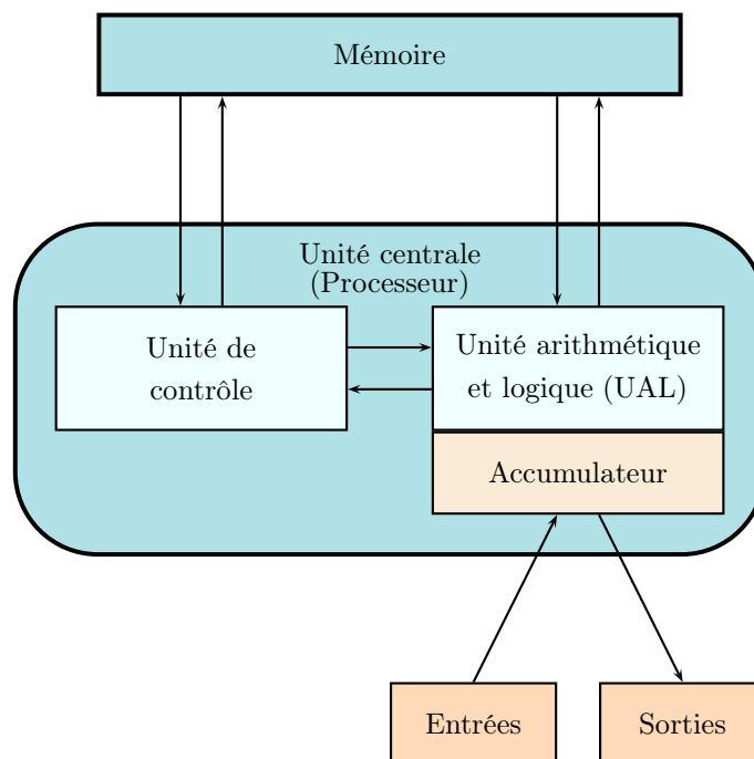
FIGURE 2.1 – Modèle d'architecture de Von Neumann
