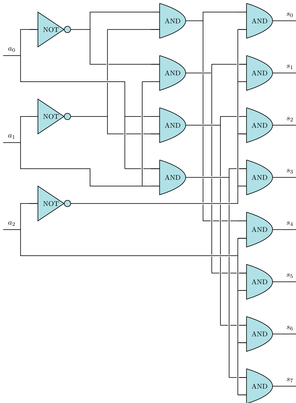
FIGURE 2.8 – Décodeur d’adresses sur 3 bits
