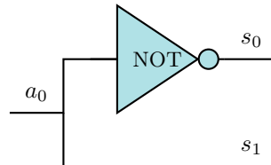
FIGURE 2.6 – Décodeur d'adresses sur 1 bit
