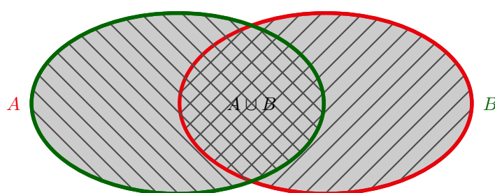
FIGURE 2.2 – Union de deux ensembles
