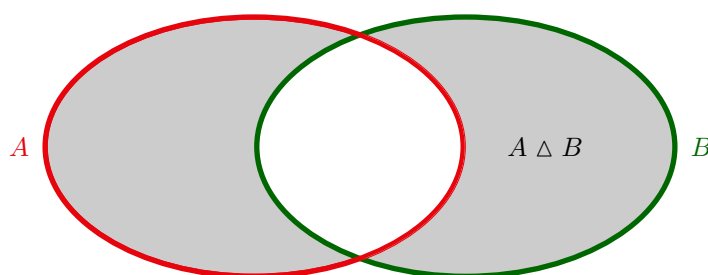
FIGURE 2.4 – Différence symétrique
