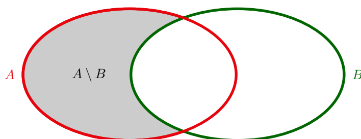
FIGURE 2.3 – Différence ensembliste
