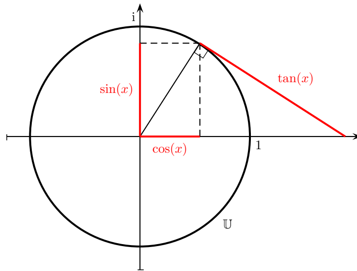
FIGURE 7.1 – Fonctions trigonométriques
