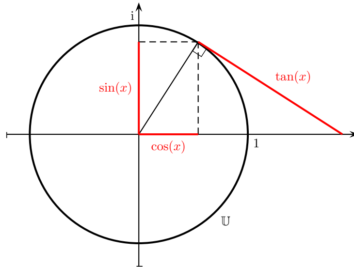
FIGURE 8.1 – Fonctions trigonométriques
